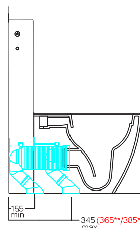
Y9D601 curva tecnica speciale tagliabile cut to size special PVC "s" trap convertor
