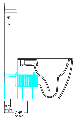
Y1CF01 curva tecnica speciale ad "L" tagliabile cut to size special PVC "L" trap convertor
