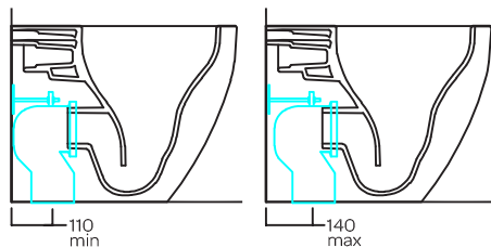
Y0EN01 curva tecnica con kit di fissaggio a parete PVC "s" trap convertor with wall fixin
