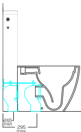
YOEN01 curva tecnica con kit di fissaggio a parete PVC "s" trap convertor with wall fixin
