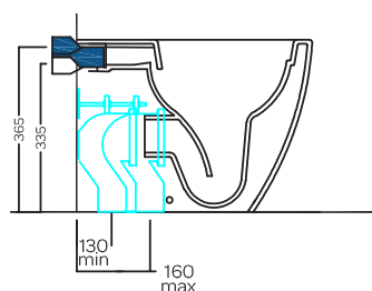
YOEN01 curva tecnica con kit di fissaggio a parete PVC "s" trap convertor with wall fixin
