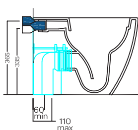
Y1CF01 curva tecnica speciale ad "L" tagliabile cut to size special PVC "L" trap convertor
