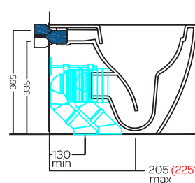
Y9D601 curva tecnica speciale tagliabile cut to size special PVC "s" trap convertor
