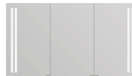
OORT 1200 mm x 677 x 158 (š x v x h) 2 zářivky 14W, vypínač, nástěnné/vestavné řešení.
