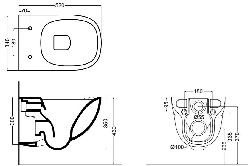
30060 vaso sospeso NORIM®_wall hung wc NORIM®
