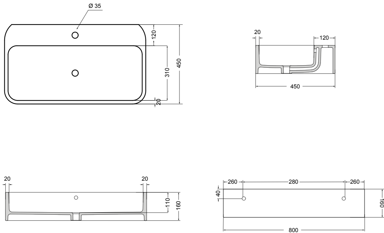
86300 lavabo appoggio/sospeso 80x45 cm_counter-top/wall-hung basin 80x45 cm
