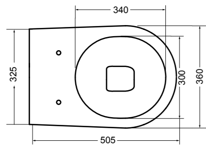
84020 bidet sospeso_wall hung bidet
